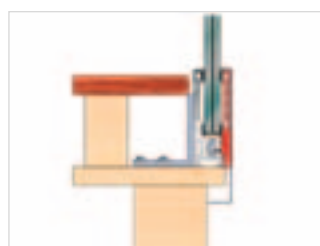
Montage auf Holz mit Konsole
