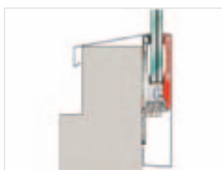
Montage mit Winkelkonsole stirnseitig
