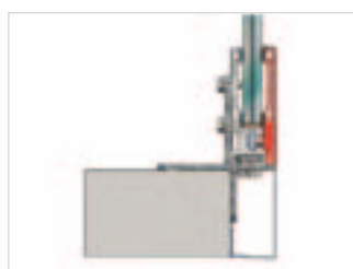
Montage mit zweiteiliger Konsole
